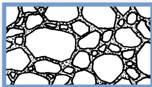
Abb. 7a: Bindemittelverbrauch durch gut abgestufte Korngrößen
