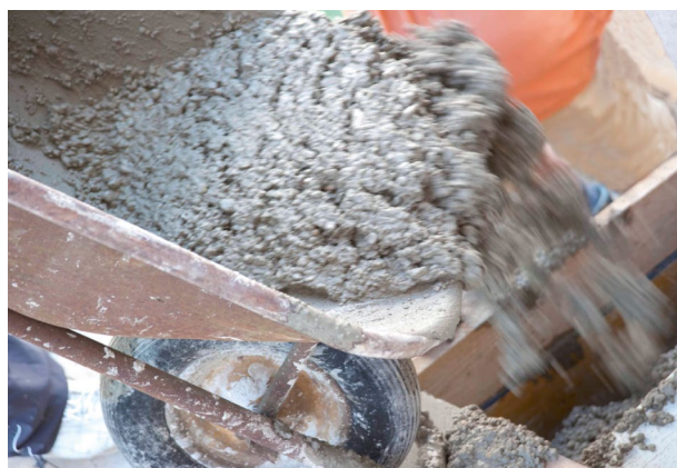
Abb. 19: Freie Fallhöhen von mehr als 1 m vermeiden
