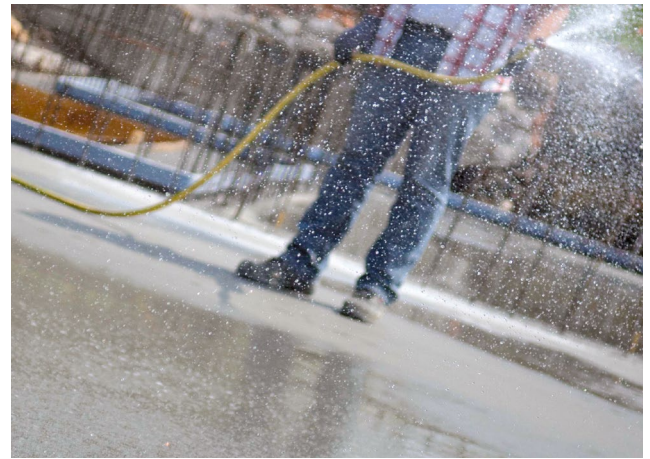
Abb. 24: Besprühen der frischen Betonoberfläche mit Wasser
